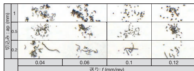
旋削
